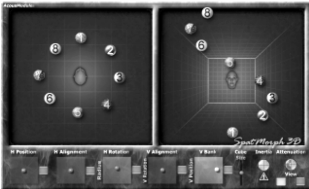
fig. 13 : SpatMorph 3D
